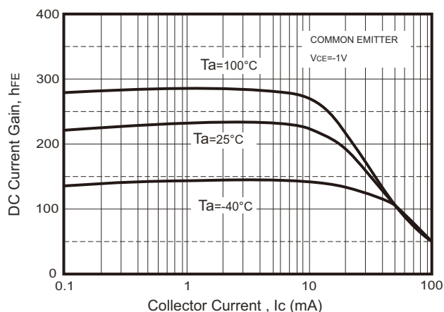
Fig.2 - h_{FE} - I_C
