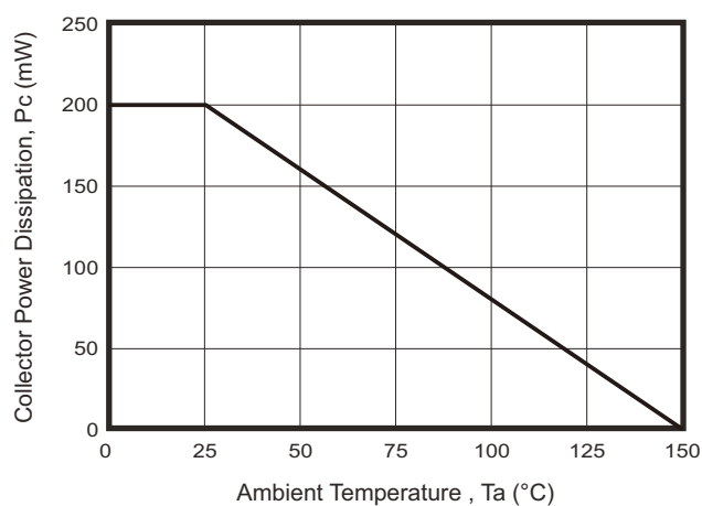
Fig. 8 - P_C - T_a
