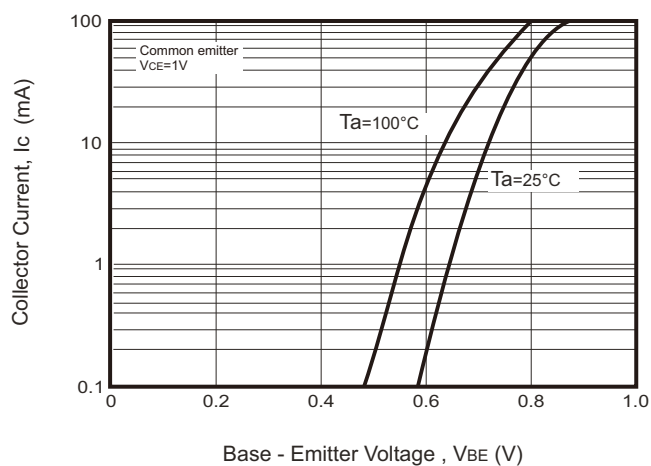
Fig. 5 - I_C - V_{BE}
